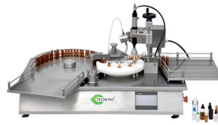
Miniblock de llenado / Engargolado para viales TECNI PAC®
